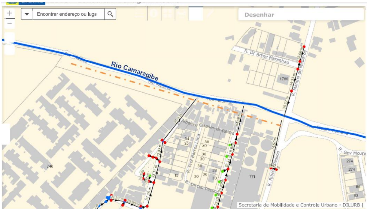
Ligação do sistema de drenagem do Residencial Marcos Freire até a Rua Ribeiro Pessoa
